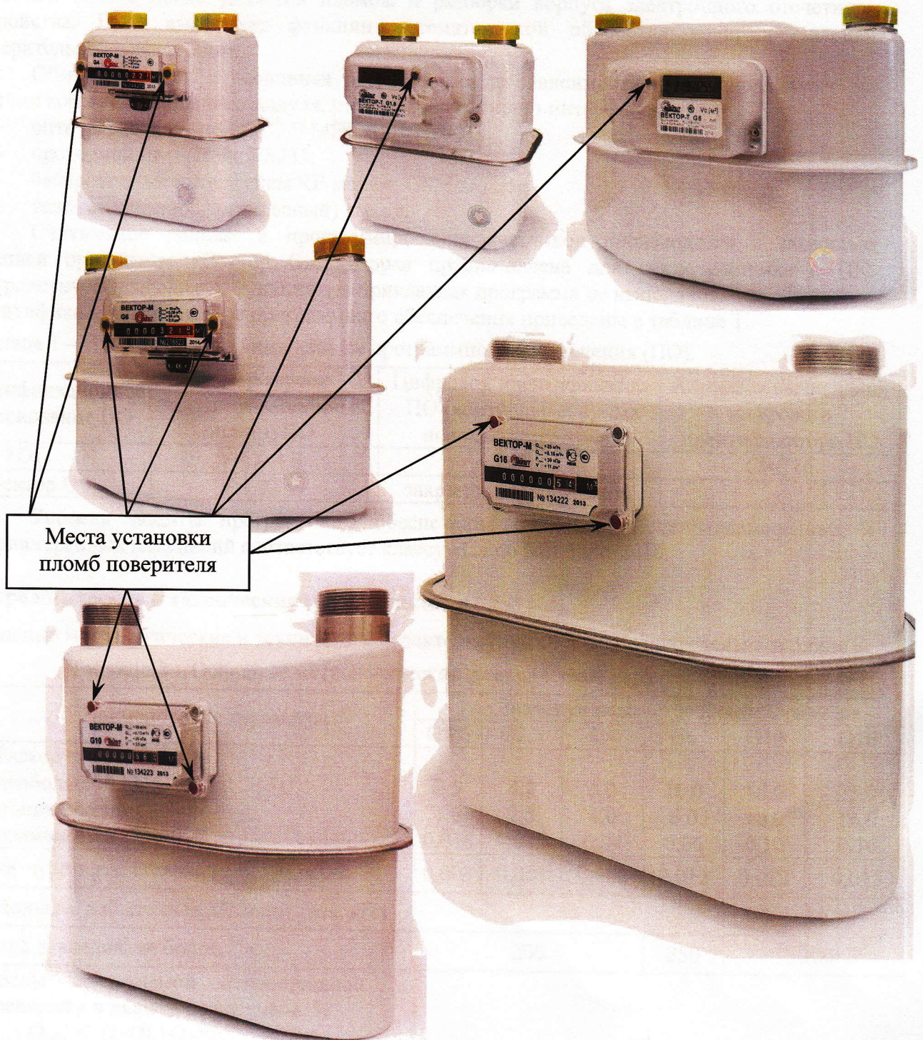
Рисунок 1 - Счетчики газа объемные диафрагменные ВЕКТОР-М/Т (G1,6; G2,5; G4; G6; G10; G16)
